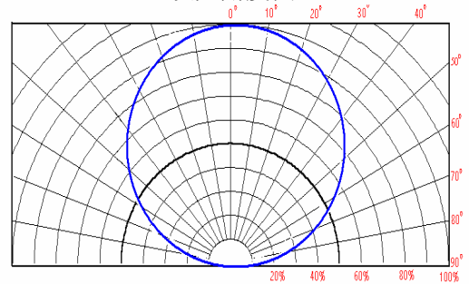
Radiation Diagram 发光角度图
