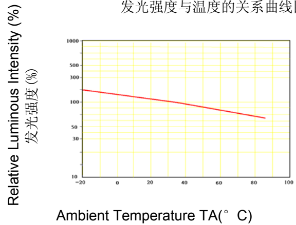
Luminous Intensity vs Ambient Temperature 发光强度与温度的关系曲线图
