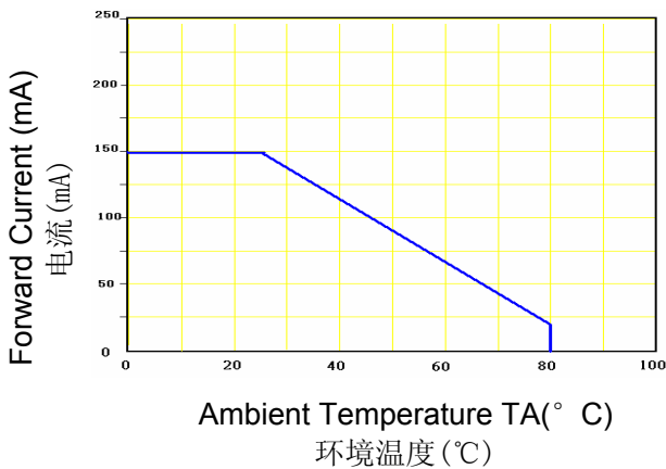
Forward Current Derating Curve 环境温度与电流的关系曲线图
