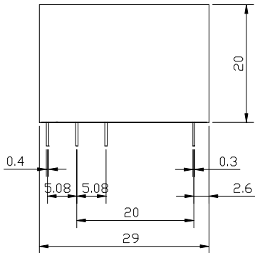
安装图
