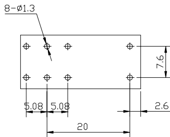
安装图
