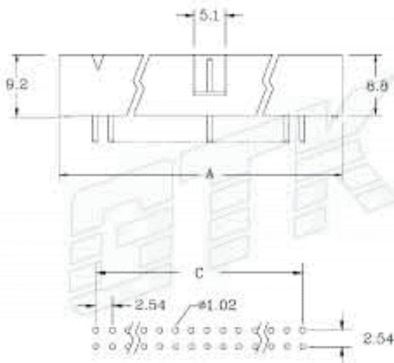
P.C.Board Layout
