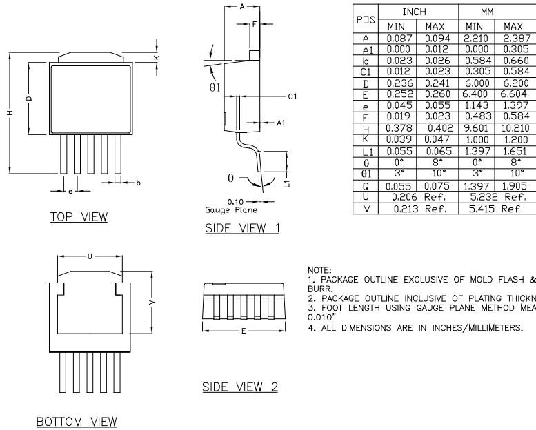
5-Pin TO-252 (D)
