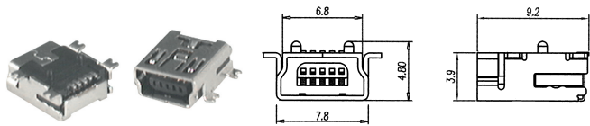
Y98905 5P MINI USB/B TYPE SOCKET (SMD TYPE)
