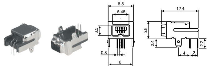
Y99045 4P MINI IEEE 1394 SOCKET
