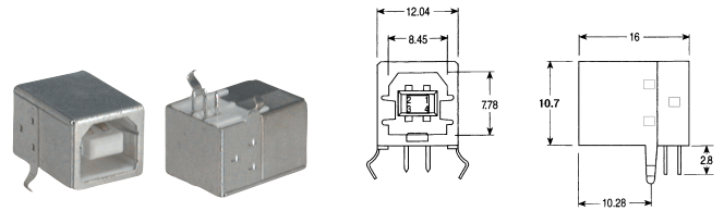
Y99011 USB/B TYPE SOCKET
