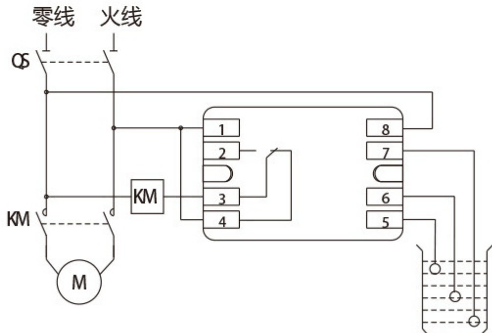
■ 220V接水方式接线图
