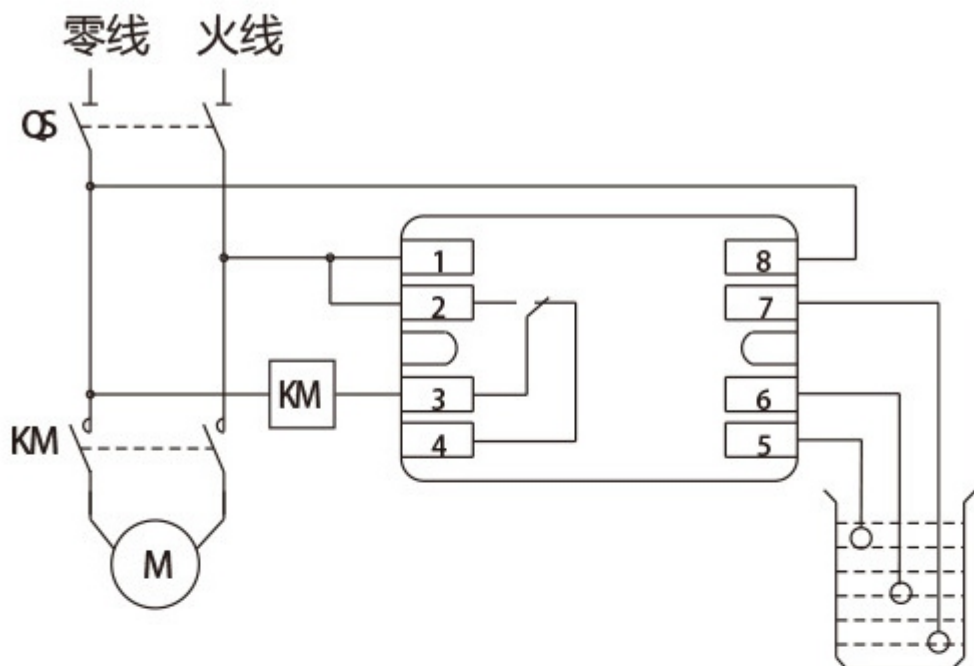
■ 220V供水方式接线图
