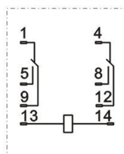
JQX-13F-MY2C
