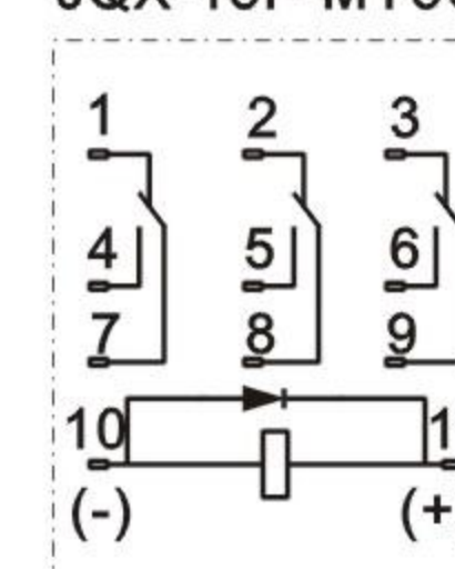
JQX-13F-MY3CD
