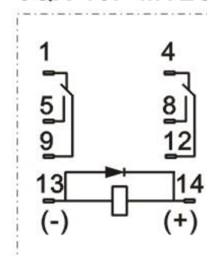
JQX-13F-MY2CD
