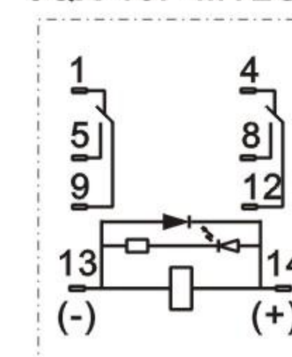
JQX-13F-MY2CLD
