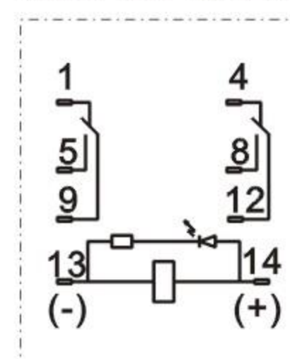
JQX-13F-MY2CL
