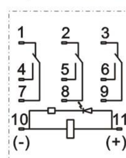
JQX-13F-MY3CL
