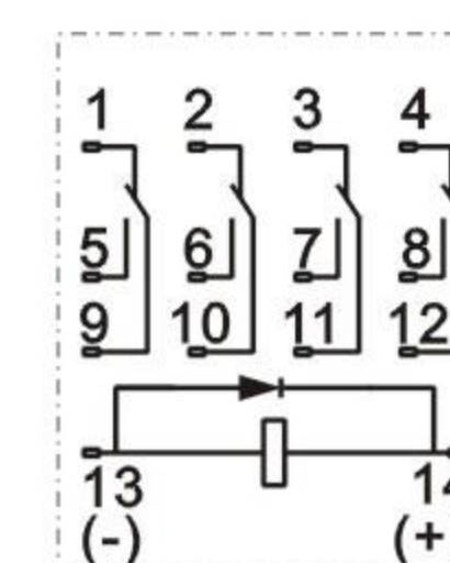
JQX-13F-MY4CD
