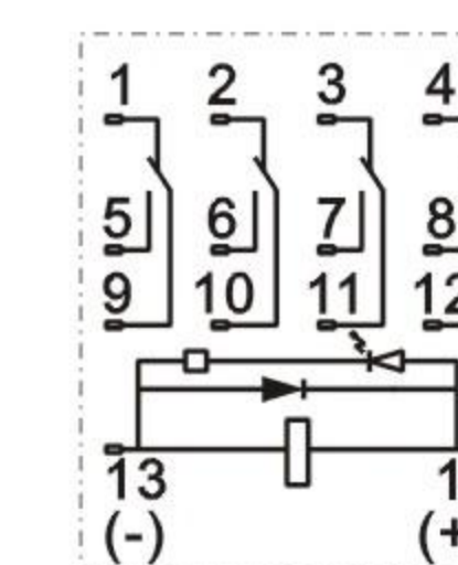
JQX-13F-MY4CLD
