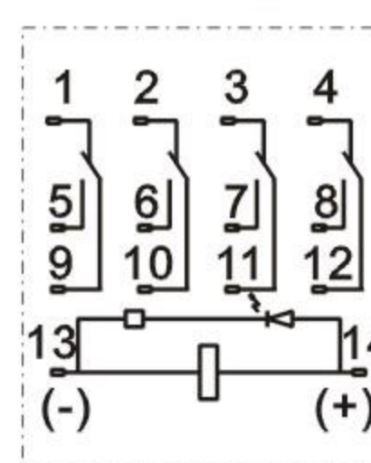
JQX-13F-MY4CL
