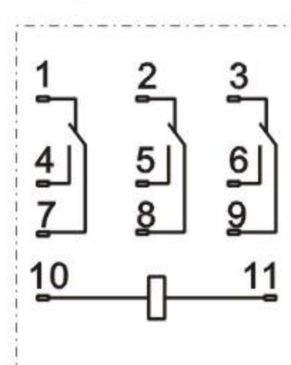
JQX-13F-MY3C
