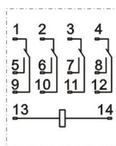
JQX-13F-MY4C
