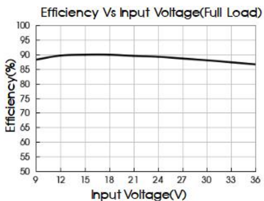
DWLD20-B2405
