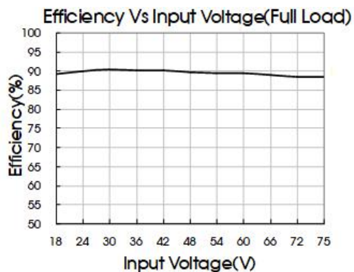
DWLD20-A4815
