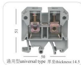
通用型universal type 厚度thickness:14.5
