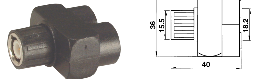
M558300 MINI BNC MALE CRIMP TYPE (RG174U/179U)
