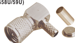
M55324 RIGHT ANGLE MINI UHF MALE CRIMP TYPE (RG58U/59U)
