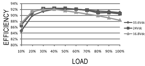
DDR-240B-24
