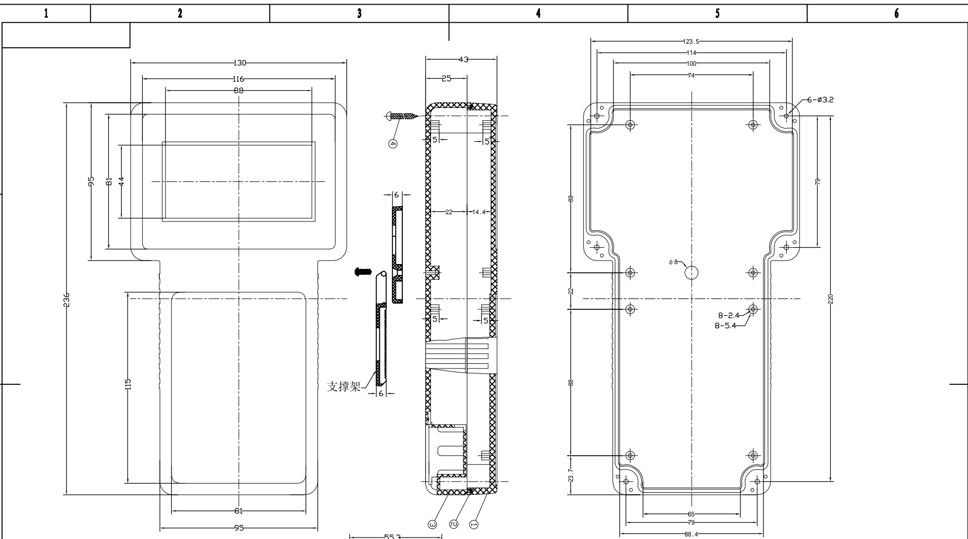
下盖正视图
