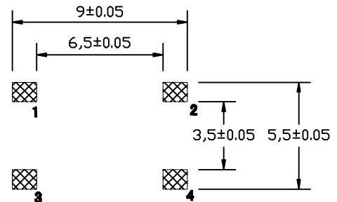
贴片尺寸 (从焊锡面看)
