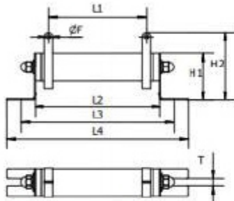
绕线型 Wirewound
