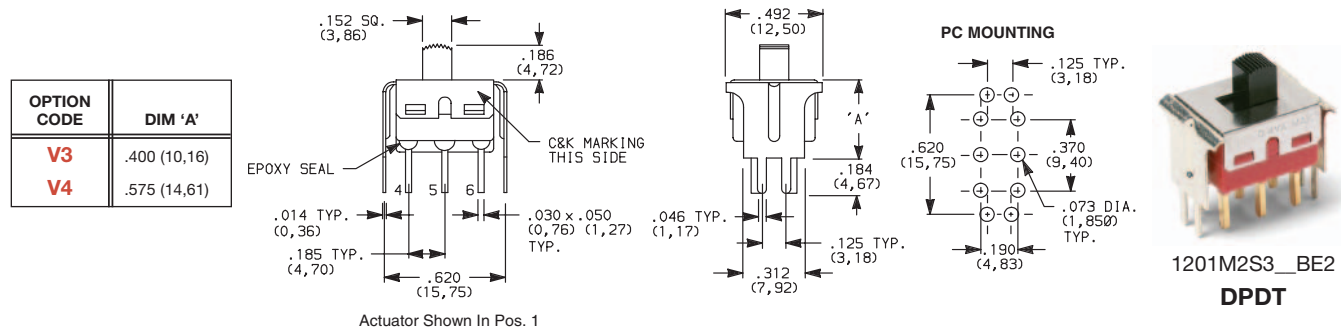
Actuator Shown In Pos. 1
