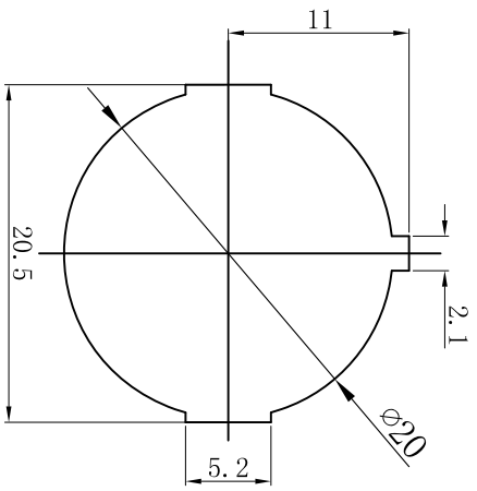
安装面板尺寸 PANEL CUT-OUT
