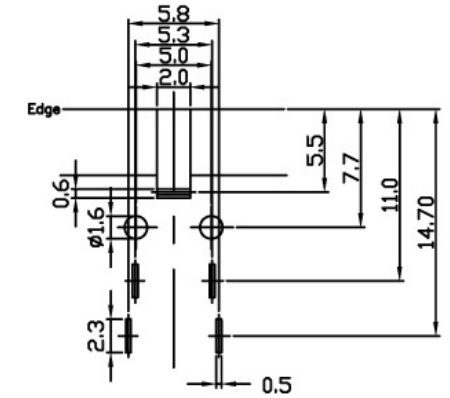
Recommend P.C.B Layout
