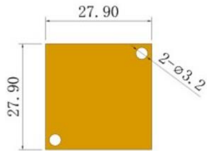
背面图 Back View
