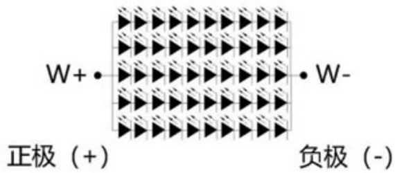
电路图 Circuit Diagram
