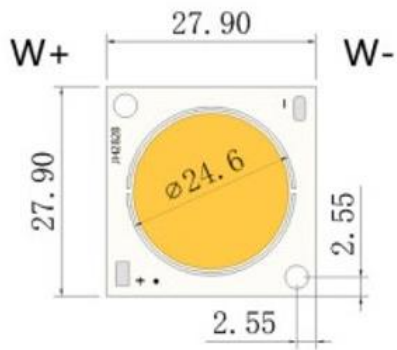
正面图 Front View
