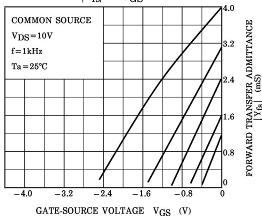
|Y_{fs}| - V_{GS}
