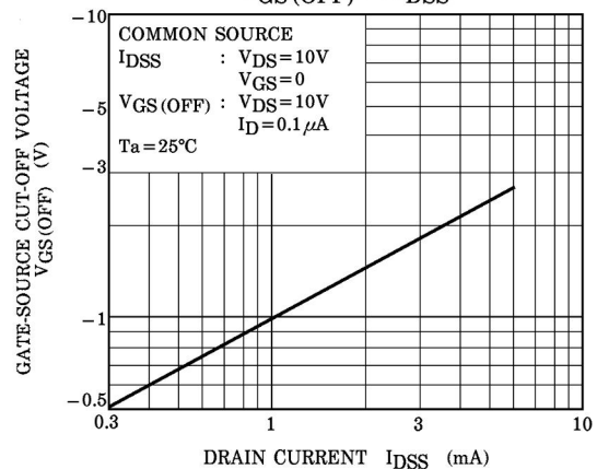
V_{GS}(\text{OFF}) - I_{DSS}
