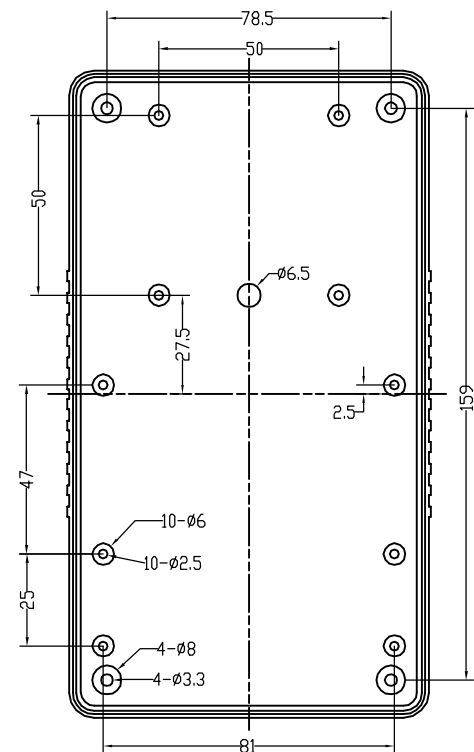
下盖正视图
