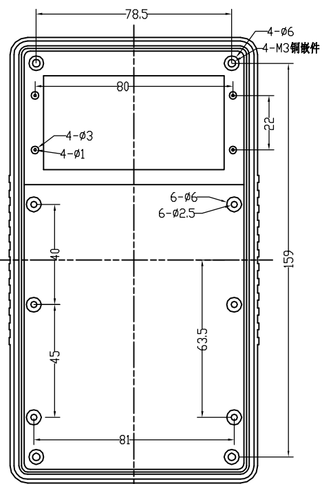
上盖底视图
