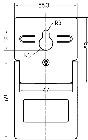
后支撑板尺寸
